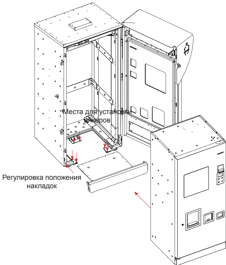
Рисунок 1 - Порядок монтажа автомата
